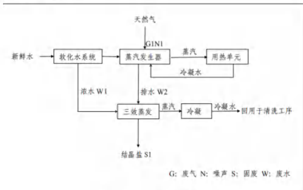
图 1 生产工艺及排污节点图
